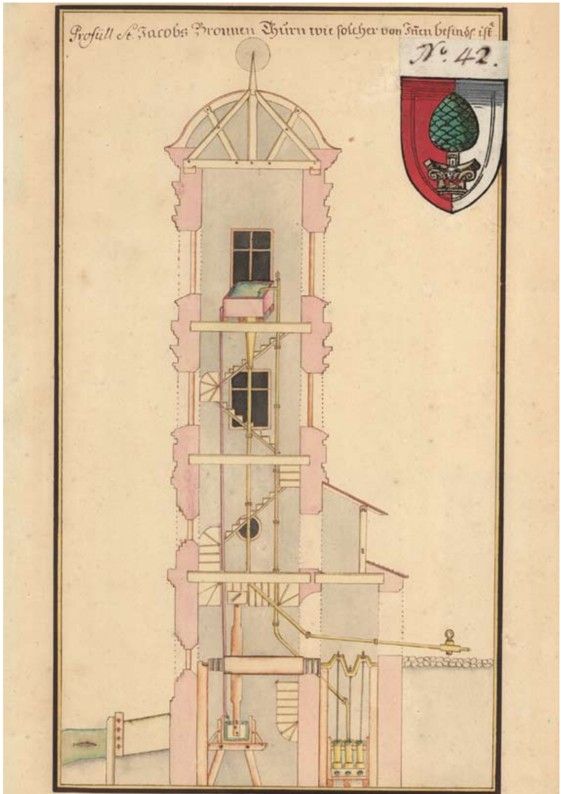
Bauzeichnung des Unteren St-Jakobs-Wasserturms in Augsburg (Zeichnung von Caspar Walter im 18. Jahrhundert)
